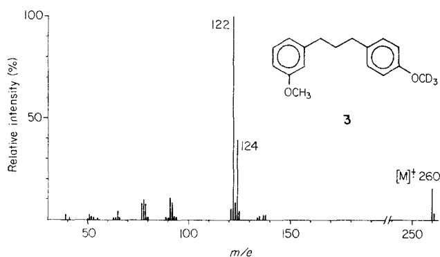
Figure 2. 70 eV mass spectrum of 1-(3-methoxyphenyl)-3-(4-trideuteromethoxyphenyl)propane ( 3 ).
