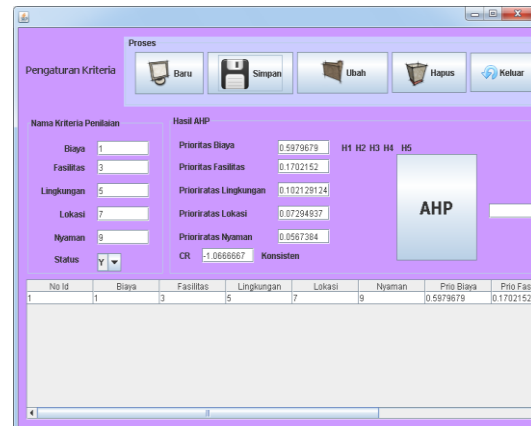
Gambar 10 Perhitungan Nilai Kriteria Pemilihan Rumah Kost
