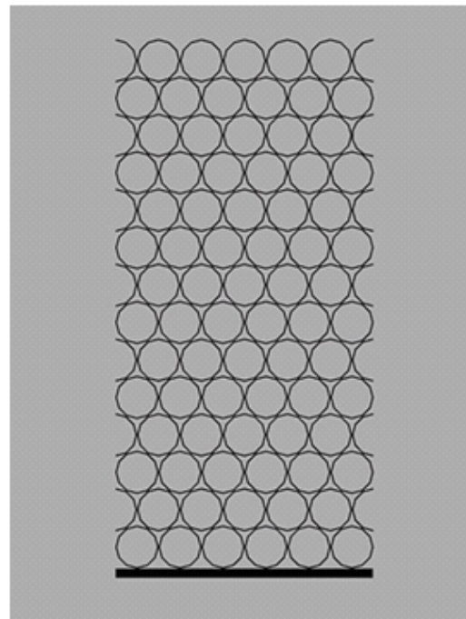
Gambar 3 Bentuk breakwater
